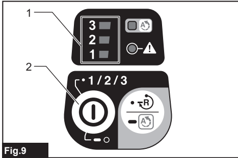
Fig.9 ► 1. Indicador de velocidad 2. Botón de encendido principal
