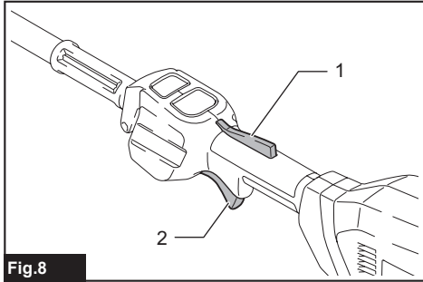
Fig.8 ► 1. Palanca de desbloqueo 2. Gatillo interruptor
