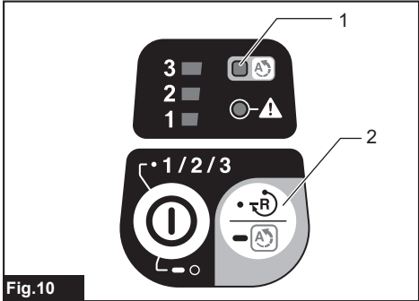
Fig.10 ► 1. Indicador de ADT 2. Botón de inversión
